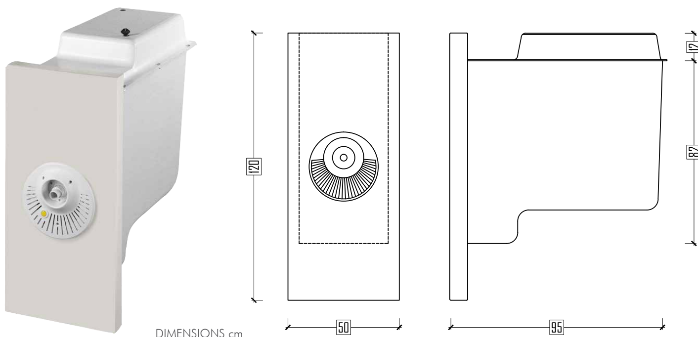
DIMENSIONS cm
